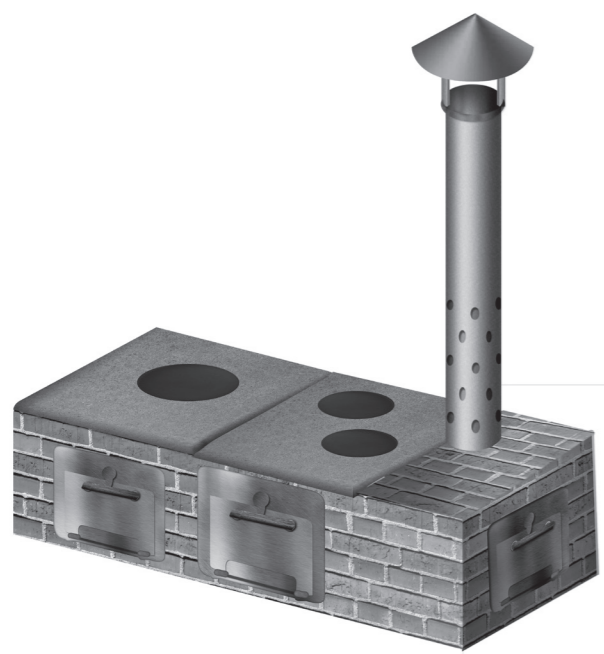
Figura 7. Perfil isométrico de la estufa SCE
