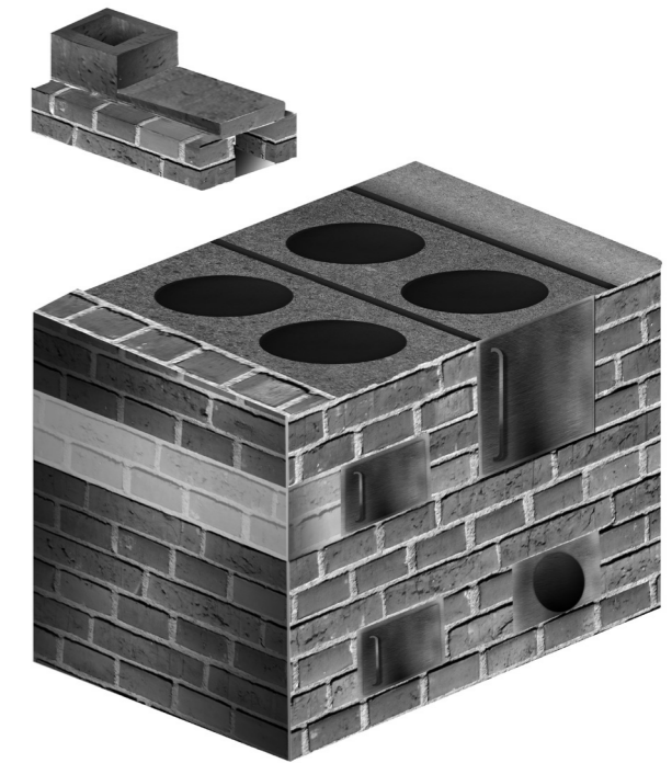
Figura 6. Perfil isométrico y cámara de combustión de la estufa FN
