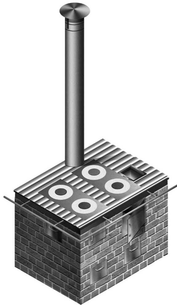
Figura 5. Perfil isométrico de la estufa Huellas
