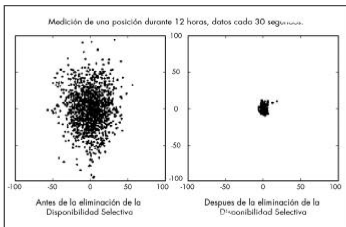
Figura 2.9: Dispersión de las posiciones obtenidas en un solo punto, antes y después de la eliminación de la Disponibilidad Selectiva, expresadas en metros.
