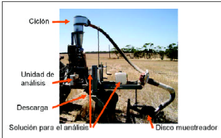
Figura 6.15: Sistema de Medición de pH Buffer y Determinación de Encalado (SpHLRMS)
