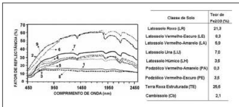
Figura 5.2: Curvas de reflectancia para diferentes tipos de suelos del Estado de San Pablo con diferentes tenores de Fe_2O_3 . FUENTE: Adaptada de Epiphânio et al. (1992).
