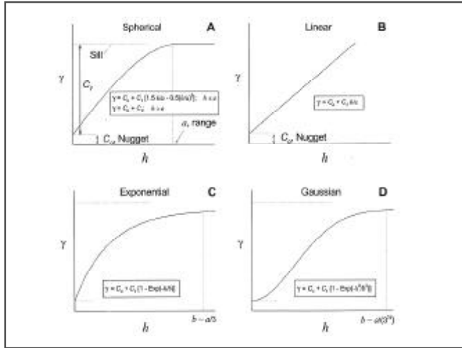
Figura 8.10: Principales modelos de variograma: (A) esférico; (B) lineal; (C) exponencial; (D) Gaussian. A su vez, en el variograma (A) se aprecian los principales componentes del mismo. Se muestran las ecuaciones que relacionan h a \gamma en cada modelo.
