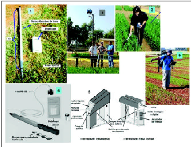
Figura 5.7: Sensores utilizados a nivel de campo para medir la radiación reflejada o emitida de doseles agrícolas: sensor cuántico (1), Spectron SE-590 (2), LAI-2000 (3 y 4), Thermopoint (5) y O FieldSpec PRO FR (6).
