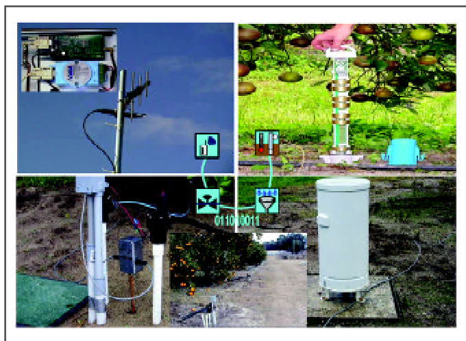
Figura 6.10: Esquema de sistema automatizado de monitoreo y aplicación de riego.
